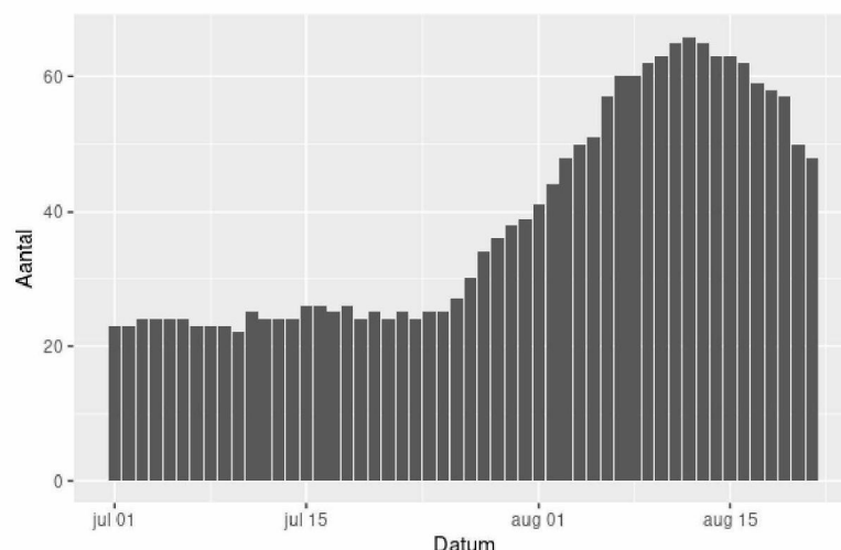
Figuur. Aantal actieve clusters per dag in verpleeghuis en woonzorg centra voor ouderen, periode 1 juli t/m 21 augustus 2020; voor recente data nog niet compleet.
